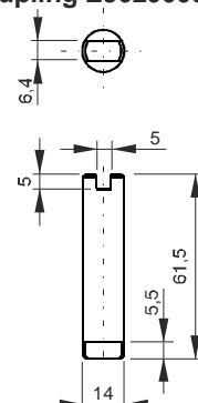
Coupling E36200005
